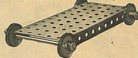
Modelo No. 00.41 Carretón plano
