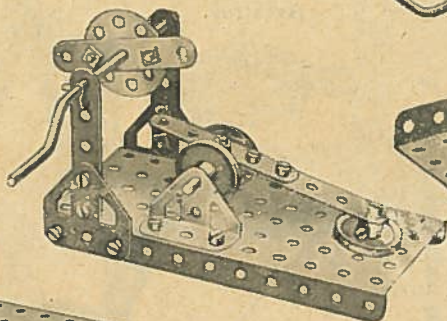
Modelo No. 00.163 Martinete
