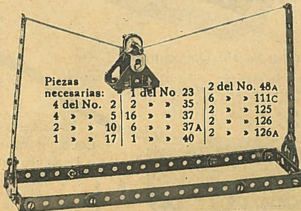
Modelo No. 0.99 Ferrocarril aéreo
