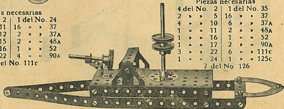
Modelo No. 0.142 Buque de Guerra
