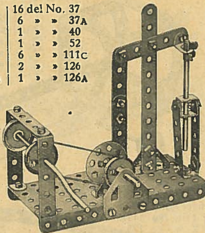
Modelo No. 0.98 Bomba
