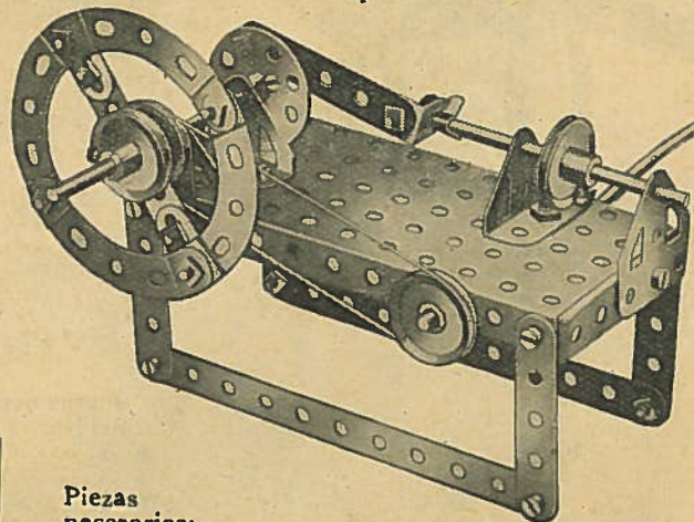
Modelo No. 0.146 Máquina horizontal
