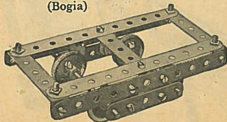
Modelo No. 00.4 Bastidor giratorio (Bogia)
