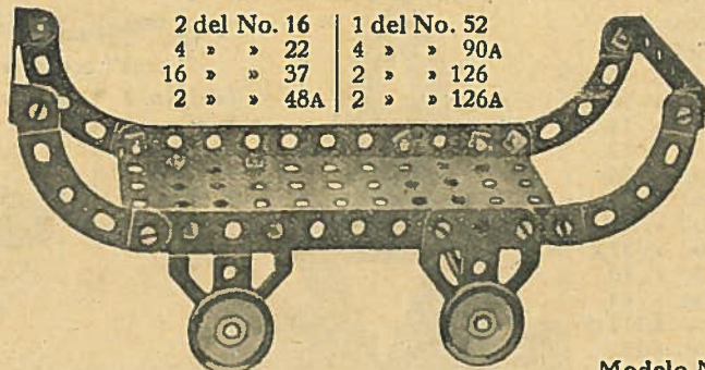
Modelo No. 03 Volquete
