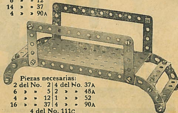
Modelo No. 0.154 Puente
