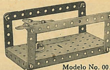
Modelo No. 00.87 Molinete
