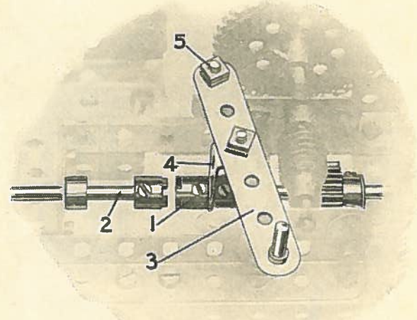
S.M. 63—DOG CLUTCH
