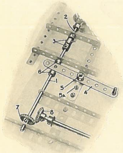
S.M. 61—DOG CLUTCH
