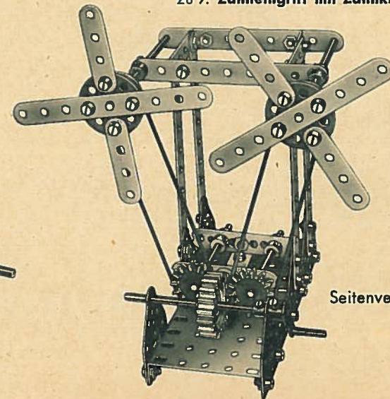
zu 9. Zahneingriff mit Zahnkranz
