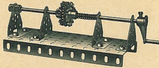
zu 7. Kupplung (axial)
