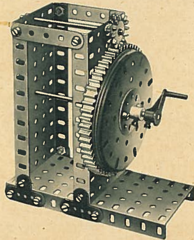
zu 9. Zahneingriff mit großem Zahnkranz
