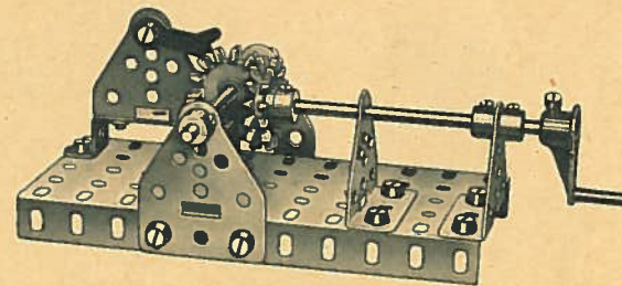
kleine Sperrklinke
