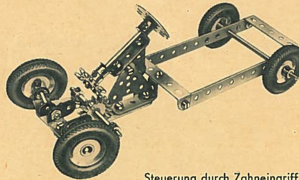
Steuerung durch Zahneingriff
