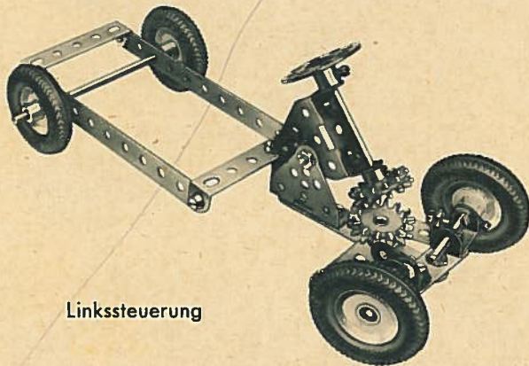
zu 3. Winkelrad
