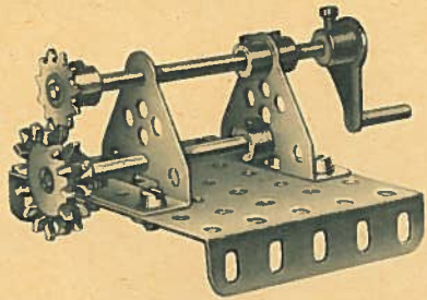
Stirneingriff mit Kettenrad Nr. 30/11
