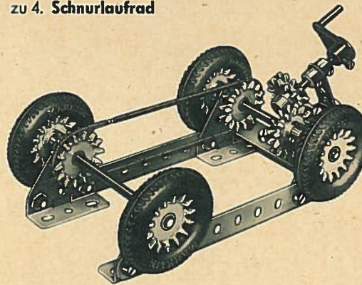
Zahnrad als Speichenrad
