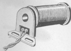
Spule mit Kern und Scheibe mit 50 cm Kabel und Steckern Nr. 0302
