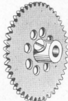
Zahnrad Nr. 025 13 Zähne " 026 10 " " 027 26 " " 027 a 19 " " 027 b 45 "
