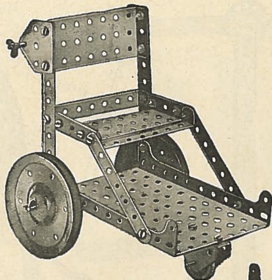
Modèle N° 74 Voiture de malade
