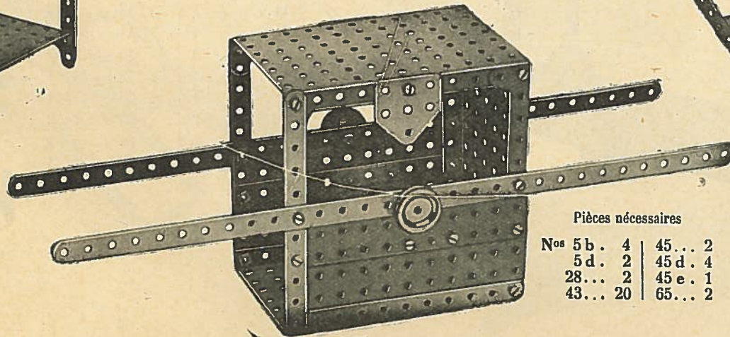
Chaise à porteur
