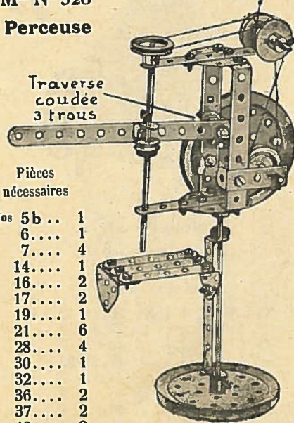
Traverse coudée 3 trous
