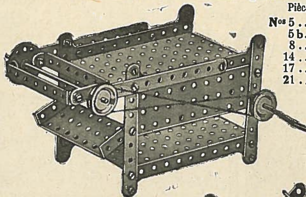
Modèle N° 206 — Hache-paille
