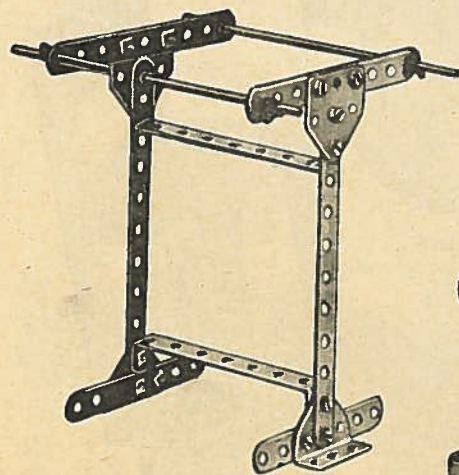
Modèle N° 93 Séchoir à linge
