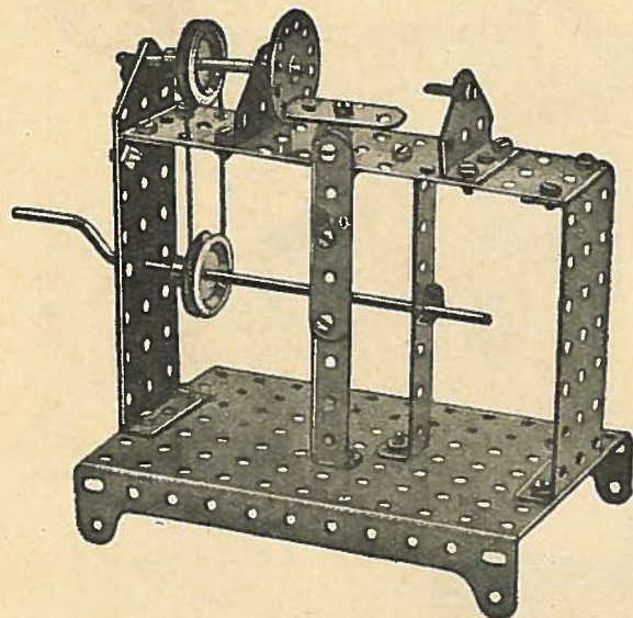
Modèle N° 90 — Tour à bois
