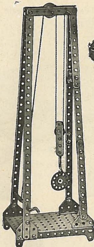
Modèle N° 207 — Palan
