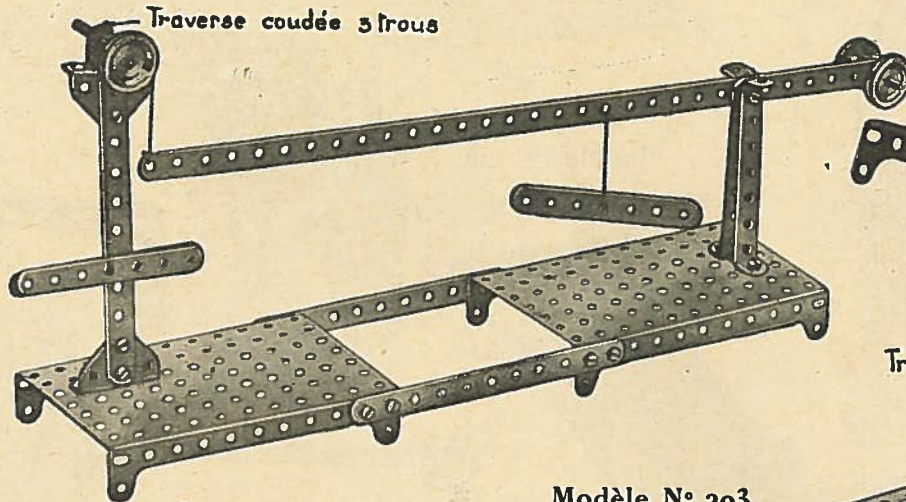
M o 201 - Levier du troisième genre
