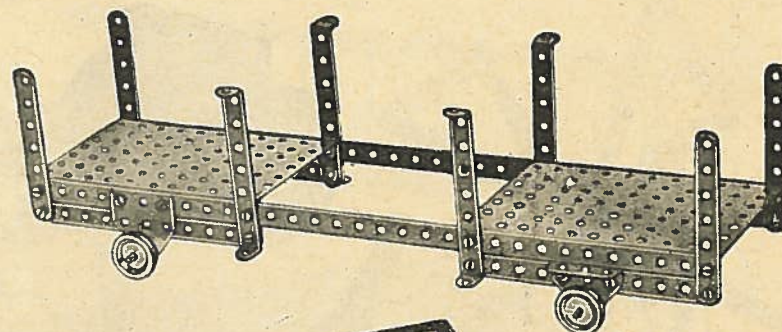
Modèle N° 234 Wagon à bois
