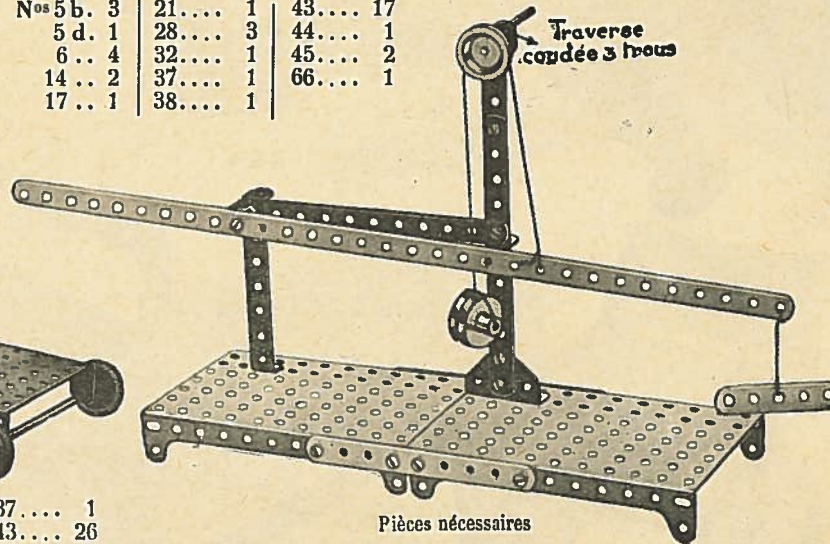
Levier du deuxième genre
