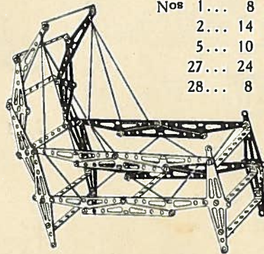
Modèle N° 86 - Berceau
