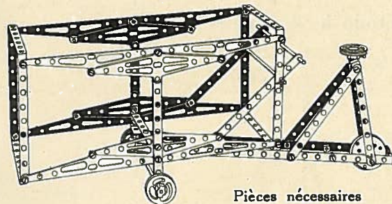
Modèle N° 81 - Triporteur
