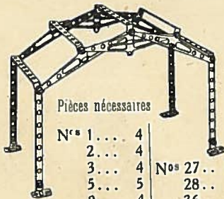
Modèle N° 14 - Hangar en voute
