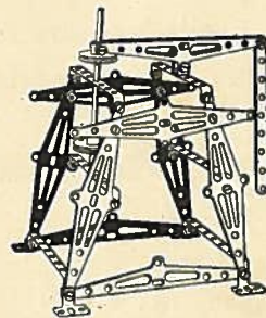
Modèle N° 32 — Martinet
