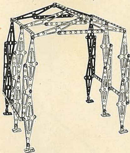
Modèle N° 131 - Hangar avec abris
