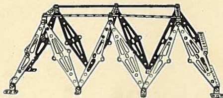
Modèle N° 26 — Passerelle
