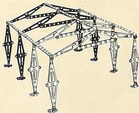
Modèle N° 132 - Hangar en longueur
