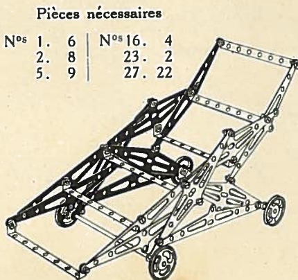
Modèle N° 80 - Voiture de malade
