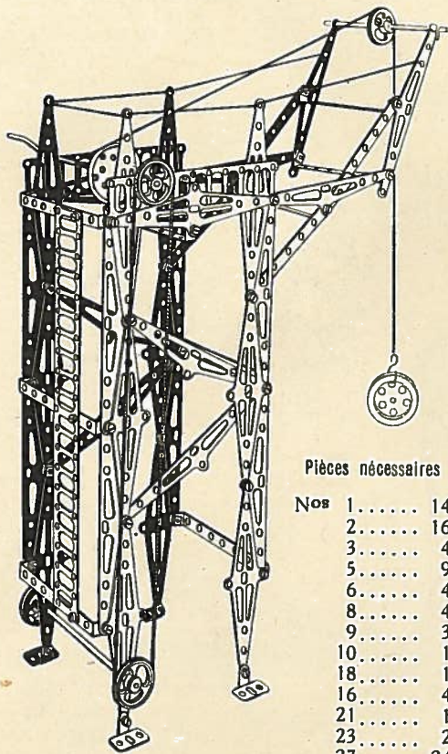
Modèle N° 101 - Monte-Charge
