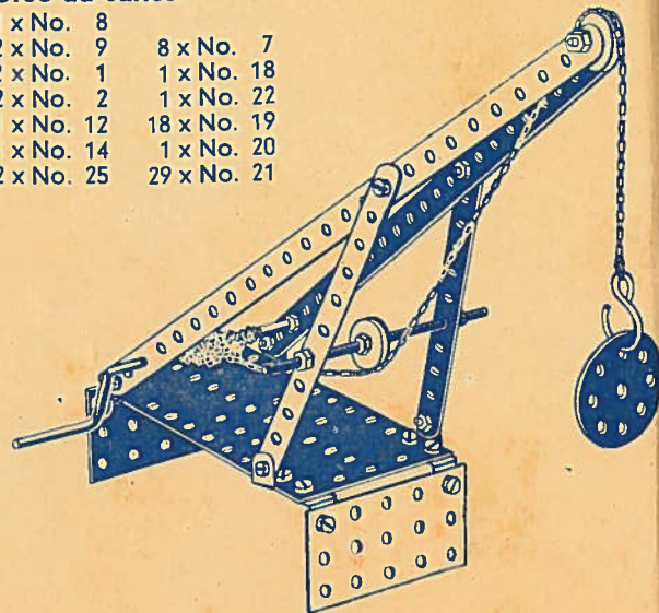
Ladekran Loading crane Grue Grúa de carga Grue da carico
