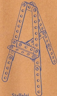
Staffelei Easel Chevalet Pilar da pintor Pilastro
