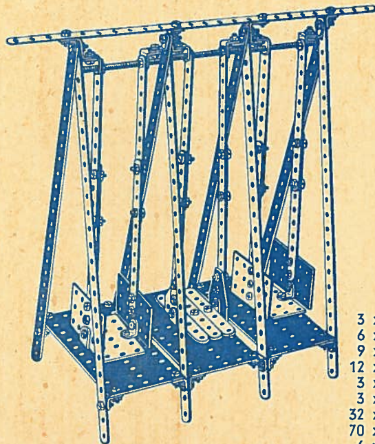
Schiffschaukel Ship-swing Balançoire à barquettes Columpio de triple asiento Alkalena a barchette
