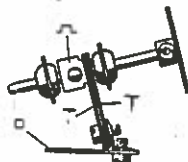
Abb. 58 a Befestigung der Steuerwelle und des Steuerrades
