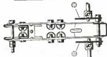
Abb. 66 a Antrieb des Selbstfahrers
