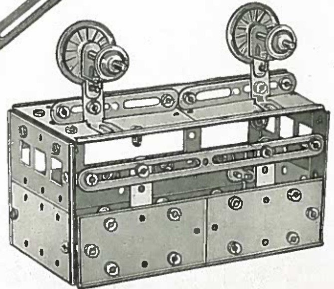
Nr. 64 Seilbahnwagen
