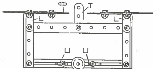
Abb. 71 a Waagebalken
