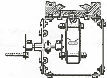
Abb. 45a Schnitt durch den Kurbelantrieb
