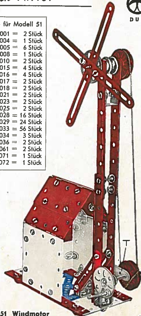
Nr. 51 Windmotor
