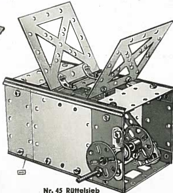
Nr. 45 Rüttelsieb
