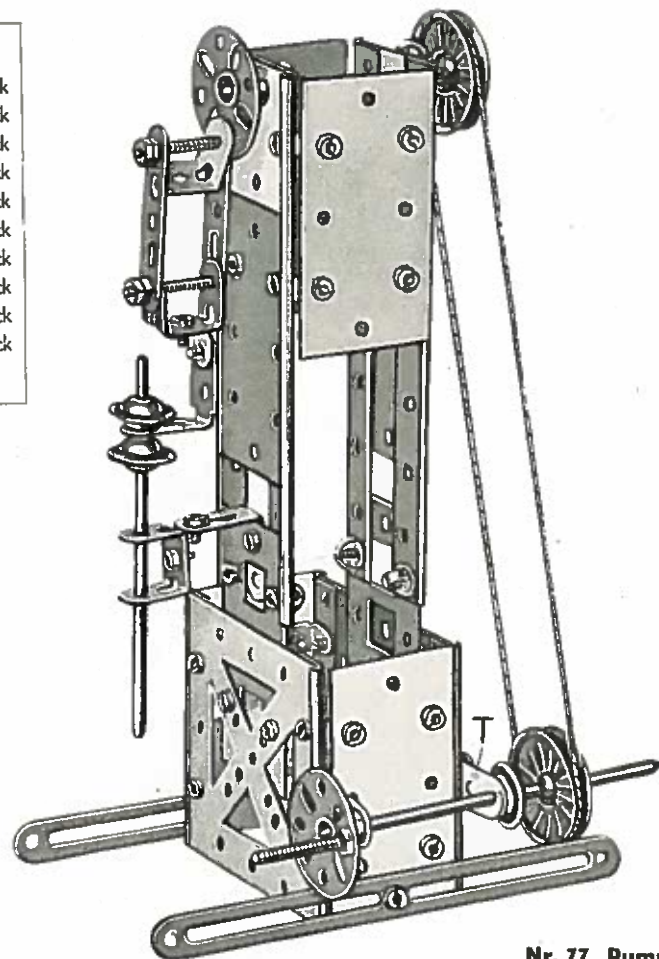
Nr. 77 Pumpe
