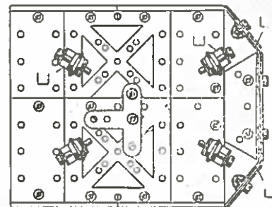
Abb. 301 b Unteransicht des Kranhausbodens
