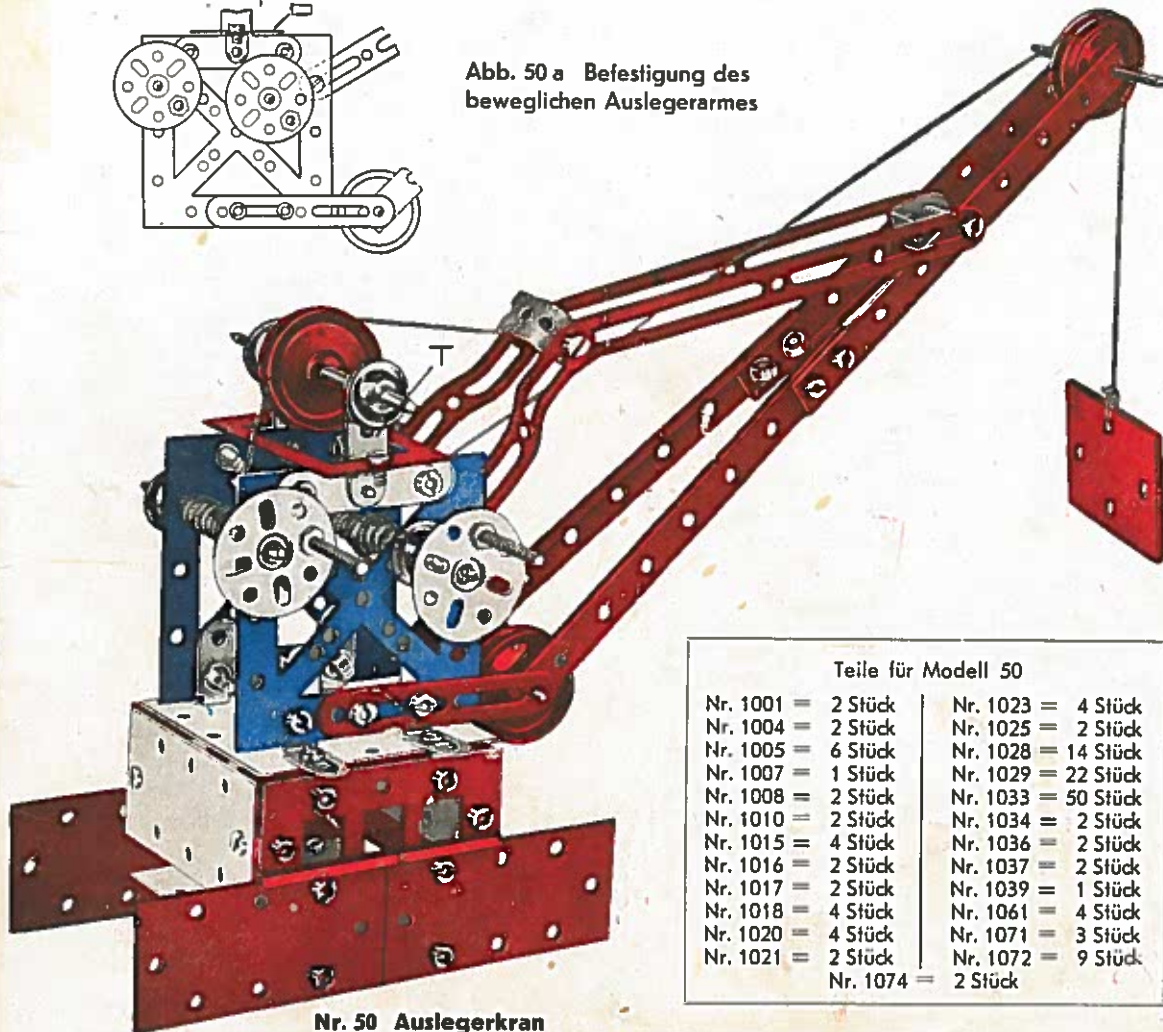
Nr. 50 Auslegerkran
