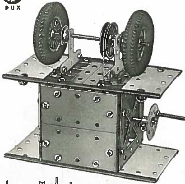
Nr. 43 Poliermaschine
