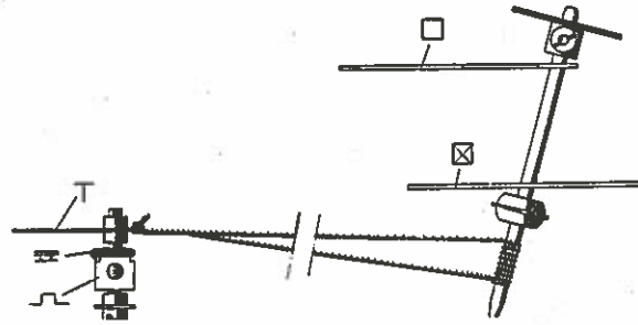
Abb. 203 b Steuerung
