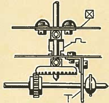
No. 97a Schnitt durch das Drehgestell Sezione del cavalletto di rotazione Section du chevrolet giratoire Tvärsnitt av vridstället.
